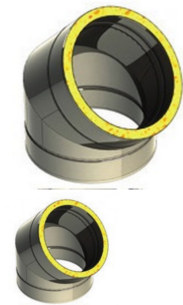
EI30 codo 45°
